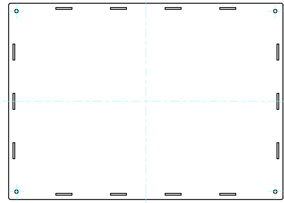
下カバー裏面 / Bottom cover Backside
