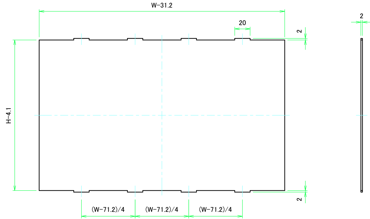
Wパネル1表面 / W Panel 1 Frontside
