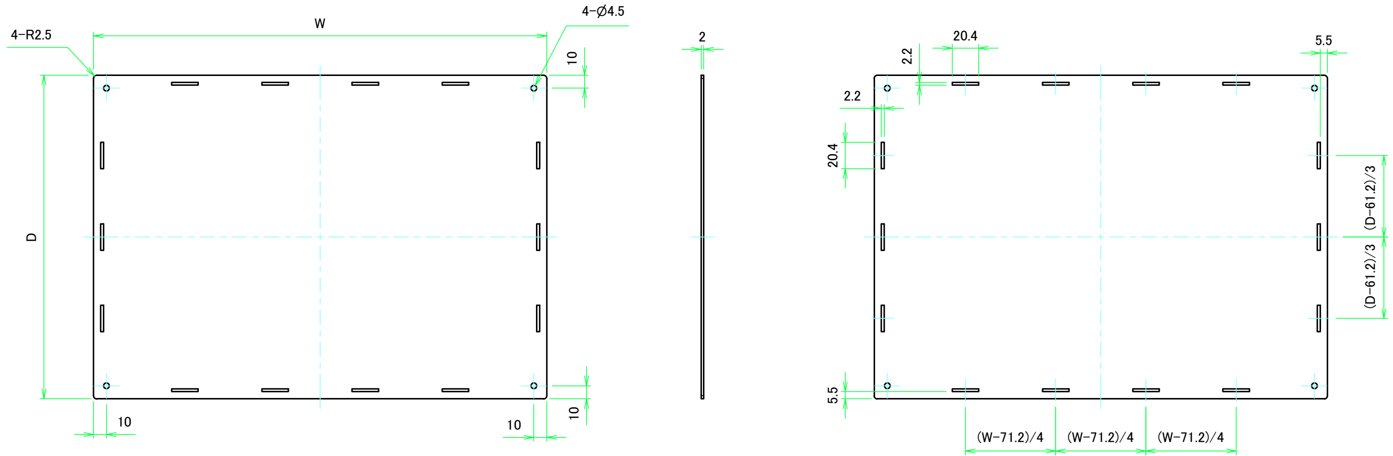
上カバー表面 / Top cover Frontside
